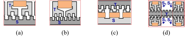
Fig. 11. Teeth variation (a) D-41 (b) D-42 (c) D-43 (d) D-44.
